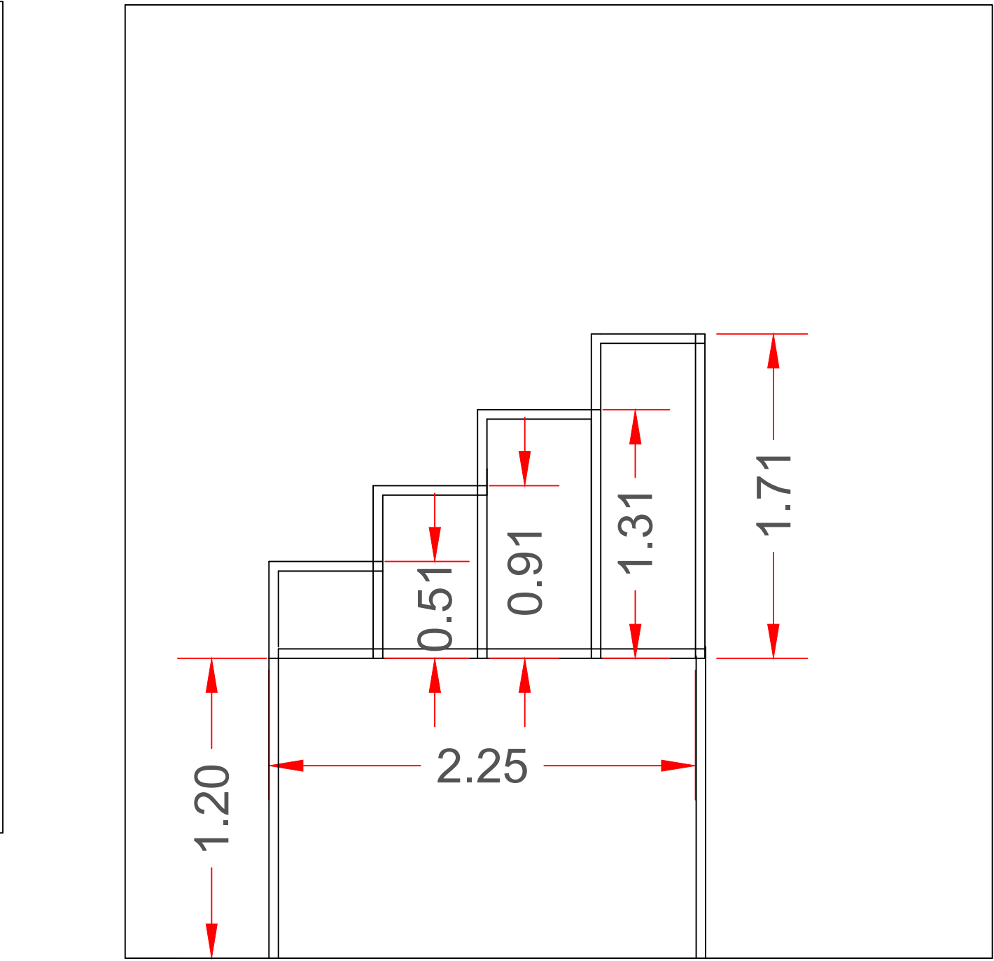
ESTRUTURA - AÇO DE CARBONO 1:100
