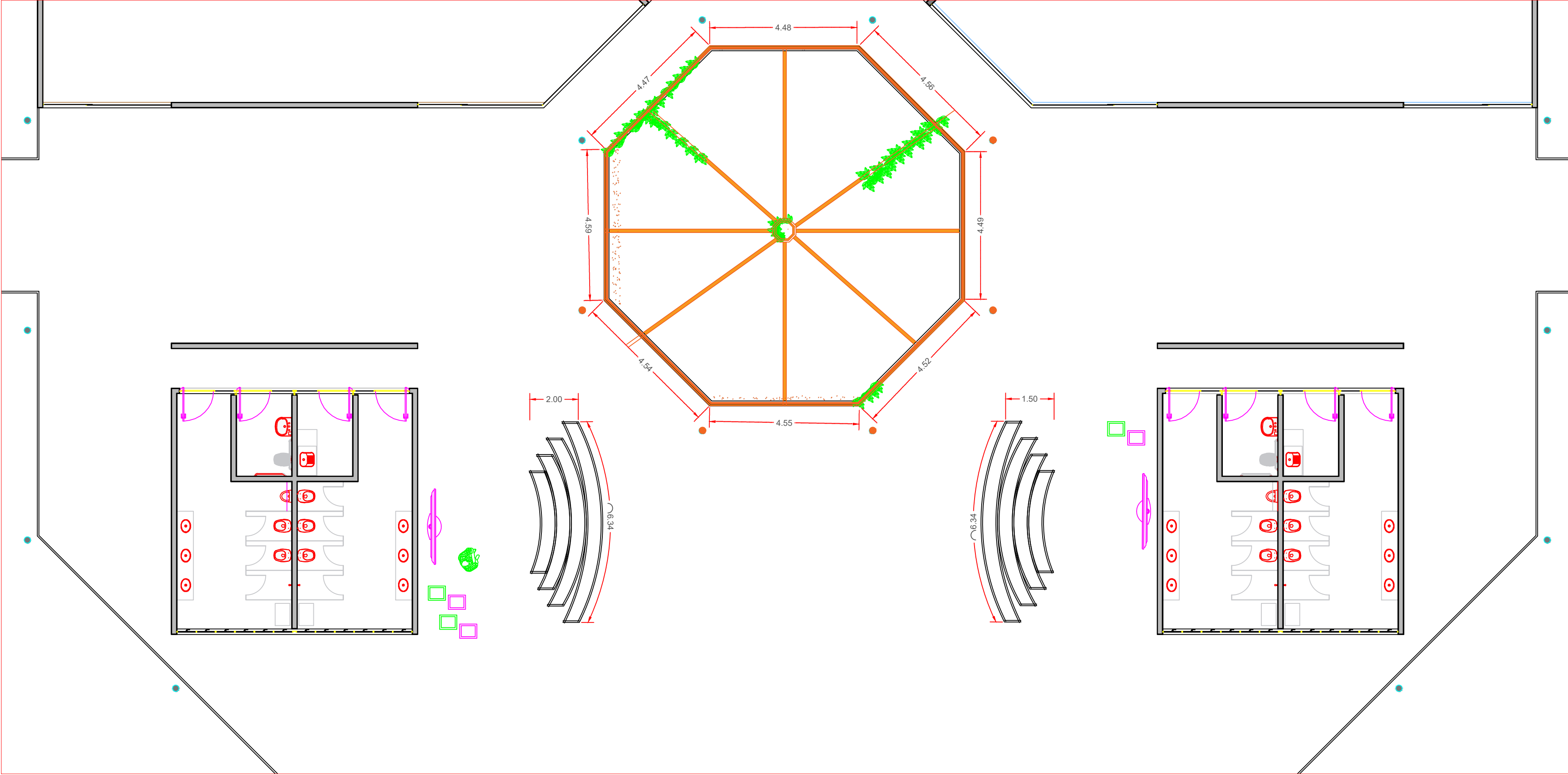
PLANTA BAIXA 1:100
